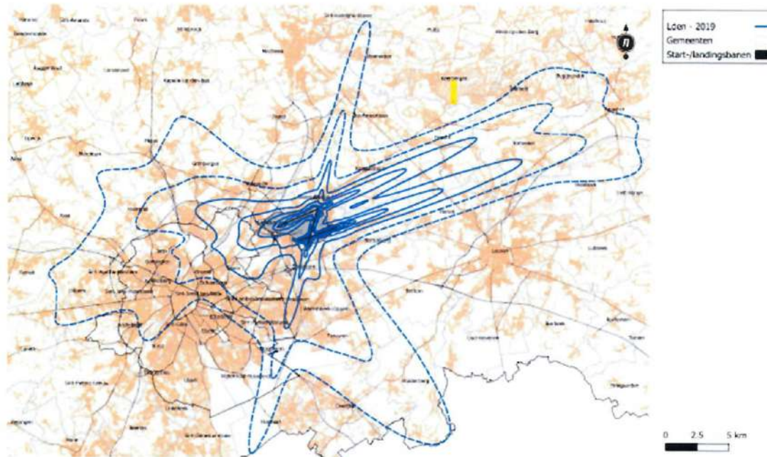
Figuur 6-27: Lden – 2019 vanaf 45 dB(A) tot 75 dB(A)
